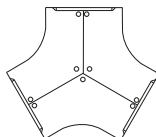
symétrique 120° 3 postes. total LG 233 PF 269 HT 74 1 poste LG 199 PF 70 HT 74
